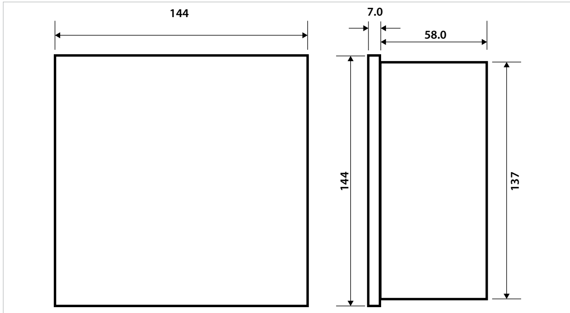
Fig. 2-8 Dimensions
