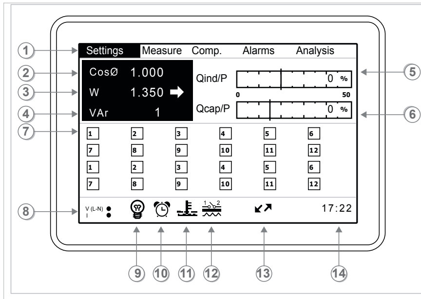
Fig. 1-2 RAPIDUS 212 R
