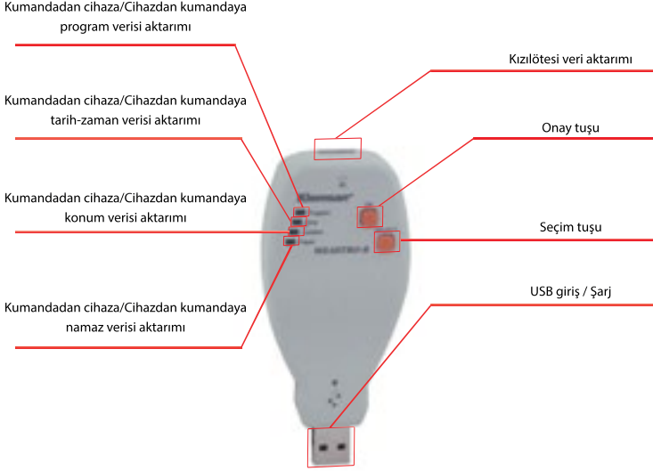
Şekil 4-1 Kumanda açıklamaları
