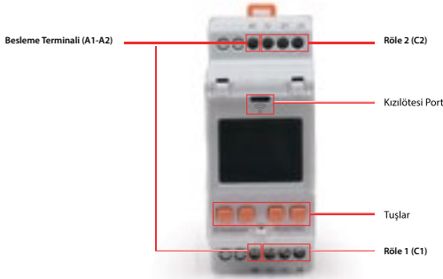
Şekil 1-2 Genel Görünüm Meastro 121, 221, 321
