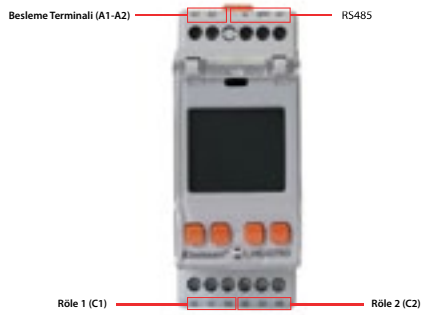
Şekil 1-3 Genel Görünüm Meastro 122, 222, 322
