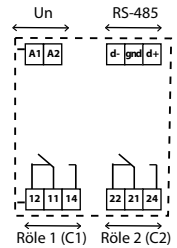
Şekil 1-6 Meastro 122, 222, 322 Baęlantı ve kablaj
